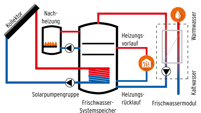
Funktionsschema COMFORT
